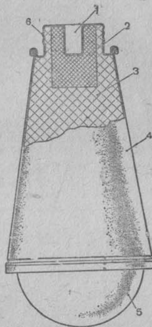
Рис. 4. Корпус гранаты (в сеч. бранном виде):
