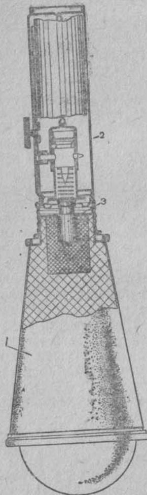
Рис. 3. Основные части ручной противотанковой гранаты РПГ-6 (вид в разрезе): 1 — корпус гранаты; 2 — рукоятка; 3 — запал
