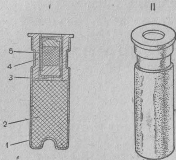
Рис. 6. Запал: I — вид в разрезе; II — наружный вид.
