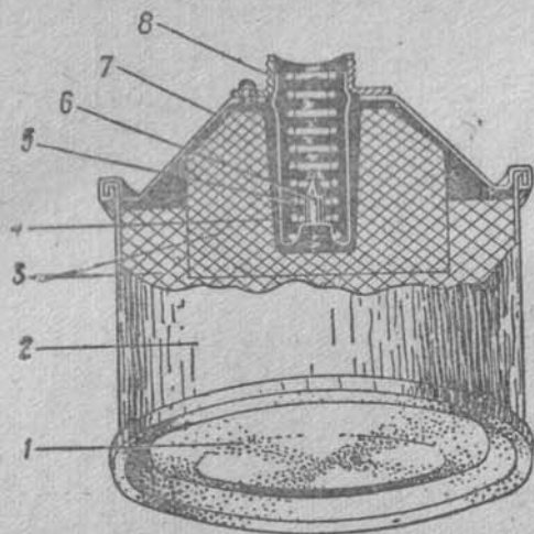
Рис. 12. Корпус гранаты:
