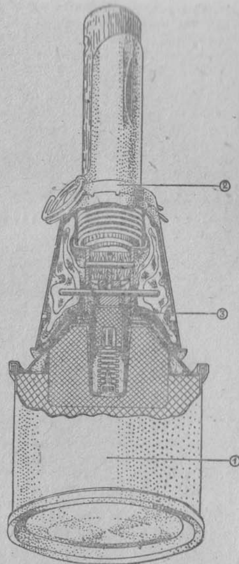
Рис. 11. Основные части ручной противотанковой гранаты обр. 1943 г. (вид в разрезе): 1 — корпус гранаты; 2 — рукоятка; 3 — запал
