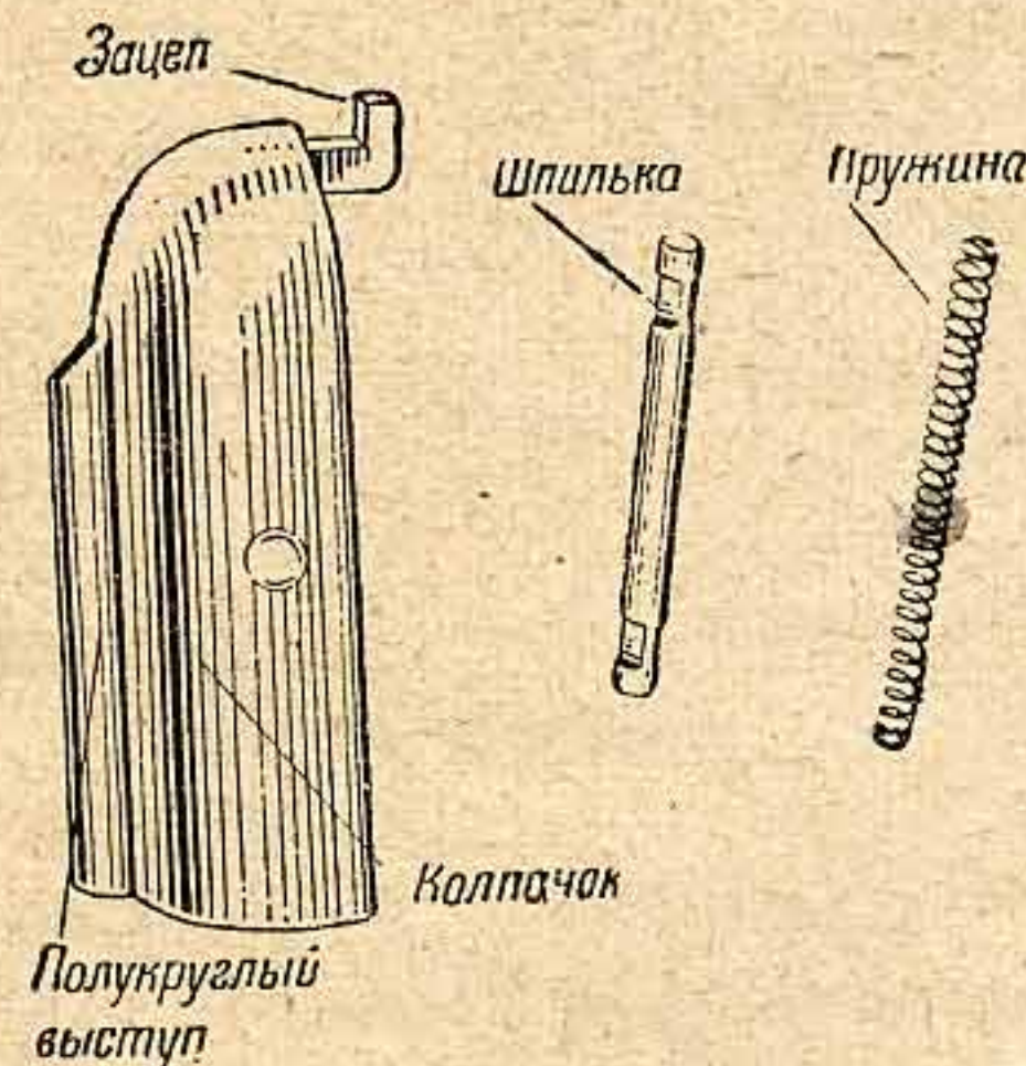
Рис. 5. Защёлка ствольной коробки
