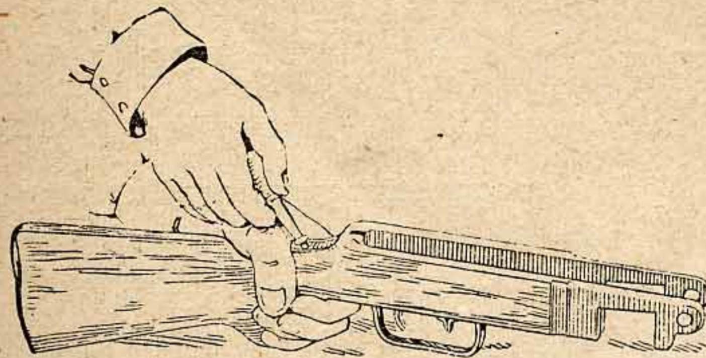
Рис. 41. Как отвинтить хвостовой винт
