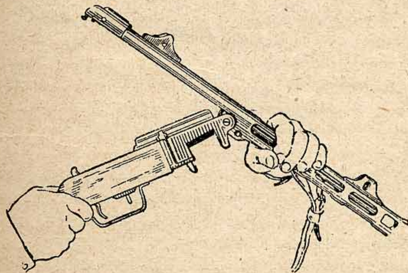
Рис. 32. Как открыть затворную коробку
