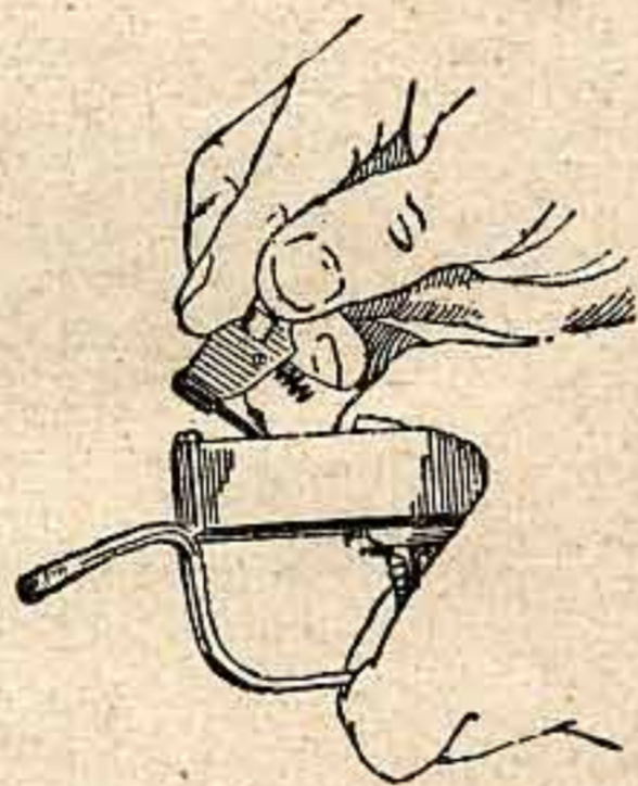
Рис. 45. Как вынуть спусковой крючок
