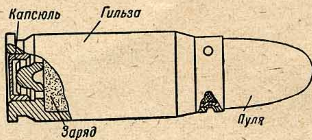
Рис. 29. Боевой патрон
