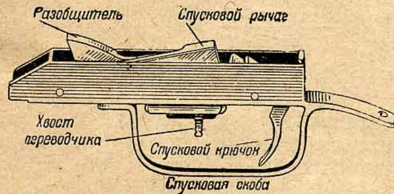
Рис. 13. Спусковая коробка со спусковым механизмом
