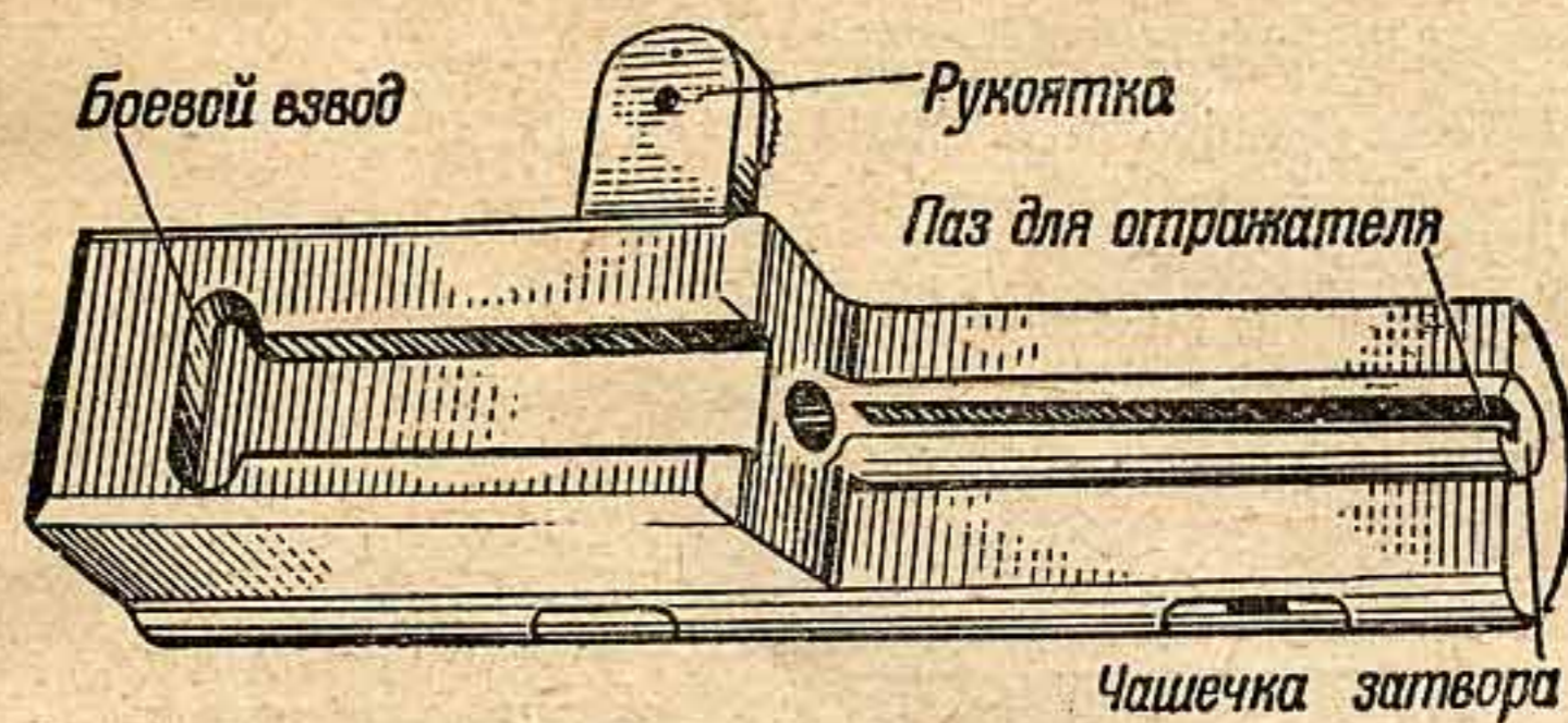
Рис. 9. Затвор
