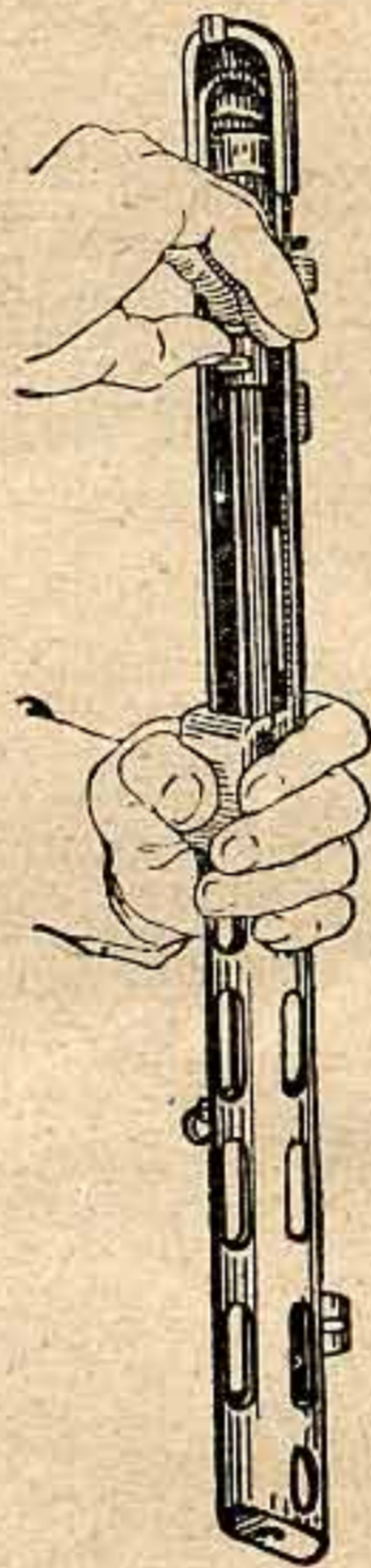
Рис. 40. Как вынуть ствол
