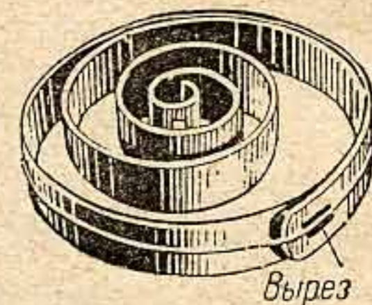
Рис. 25. Пружина магазина
