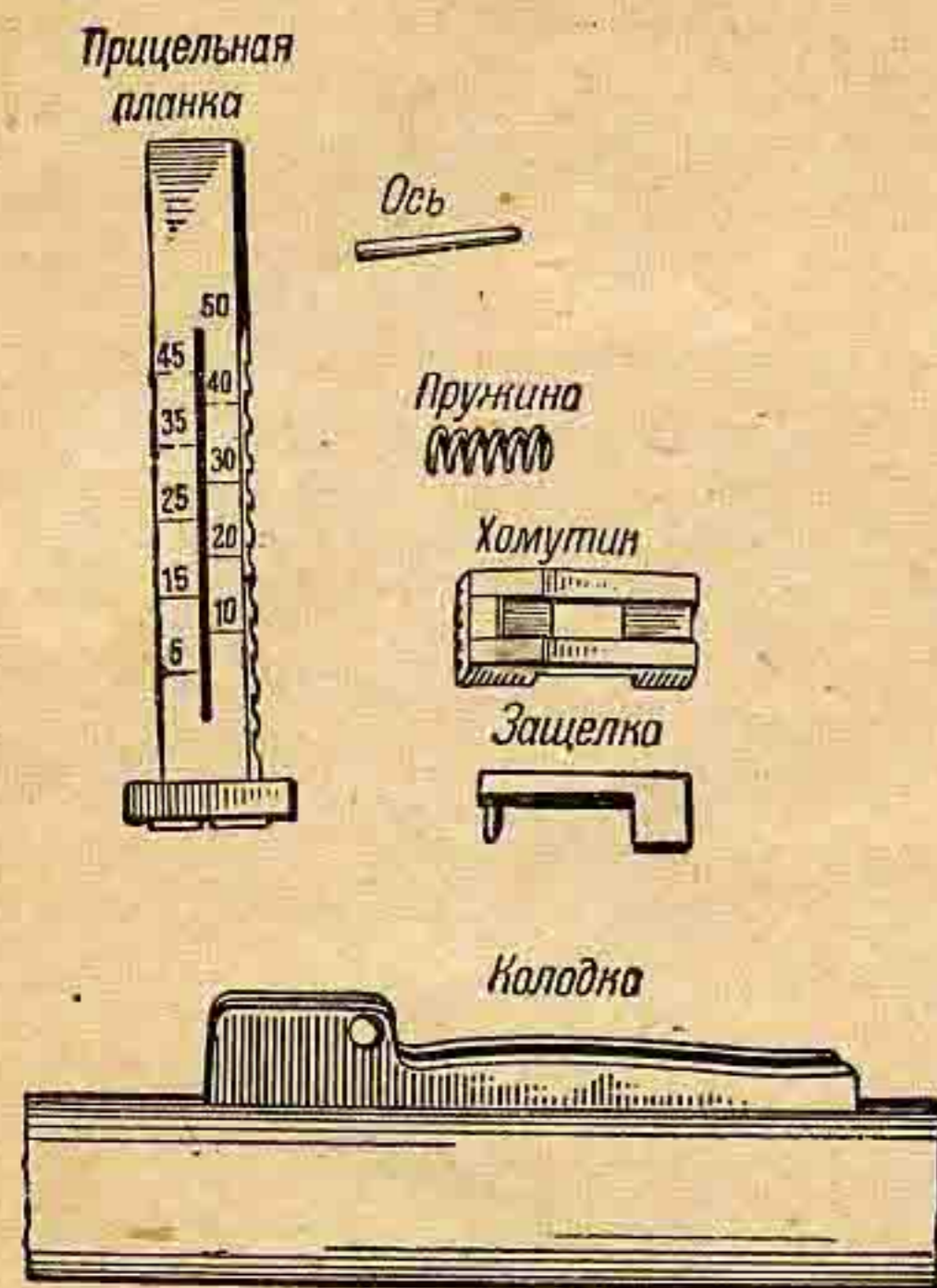
Рис. 7. Секторный прицел
