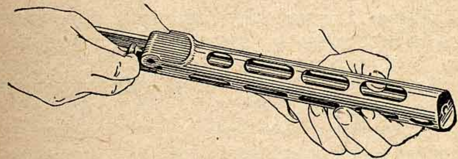
Рис. 50. Как вставить ствол
