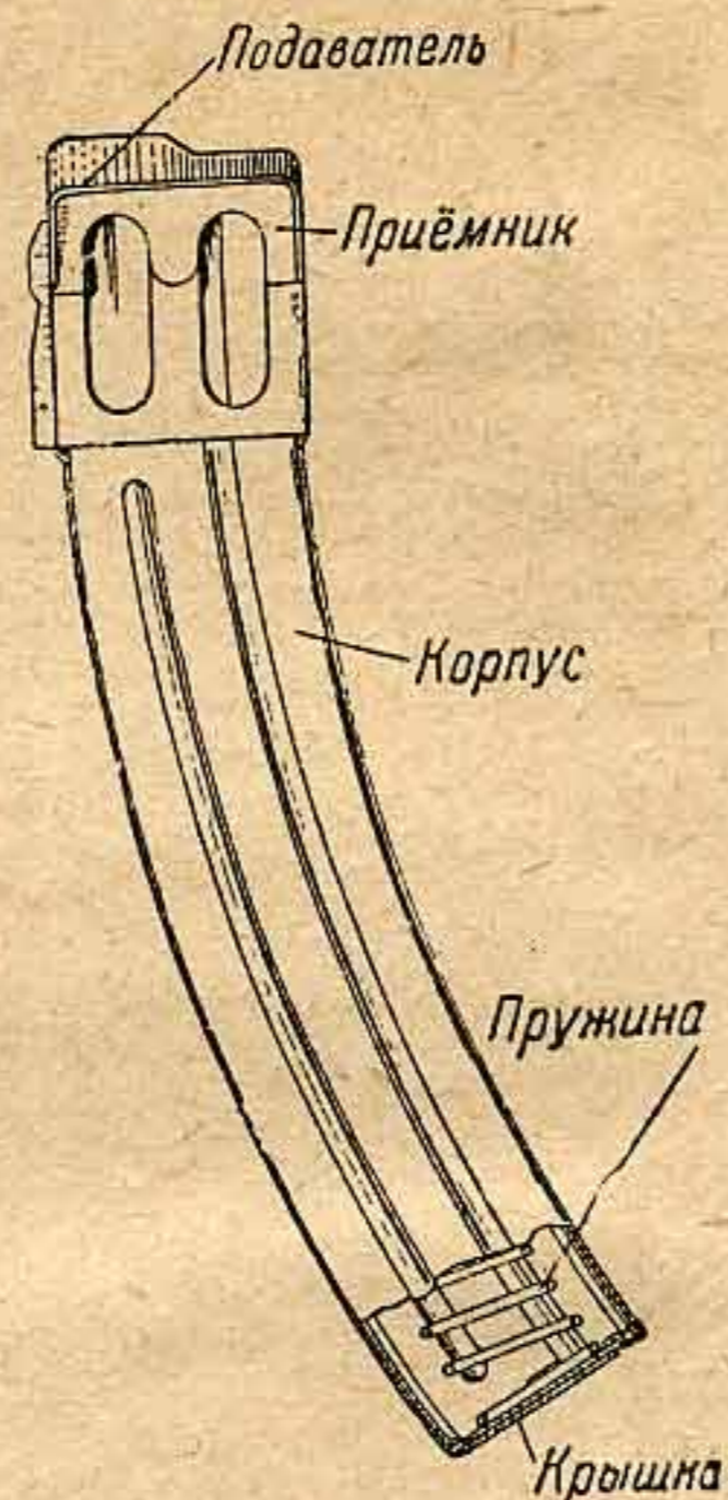
Рис. 27. Коробчатый магазин
