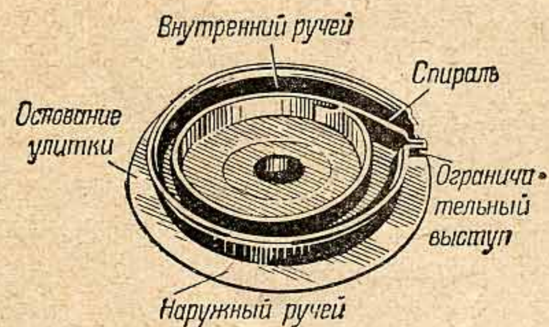
Рис. 23. Улитка
