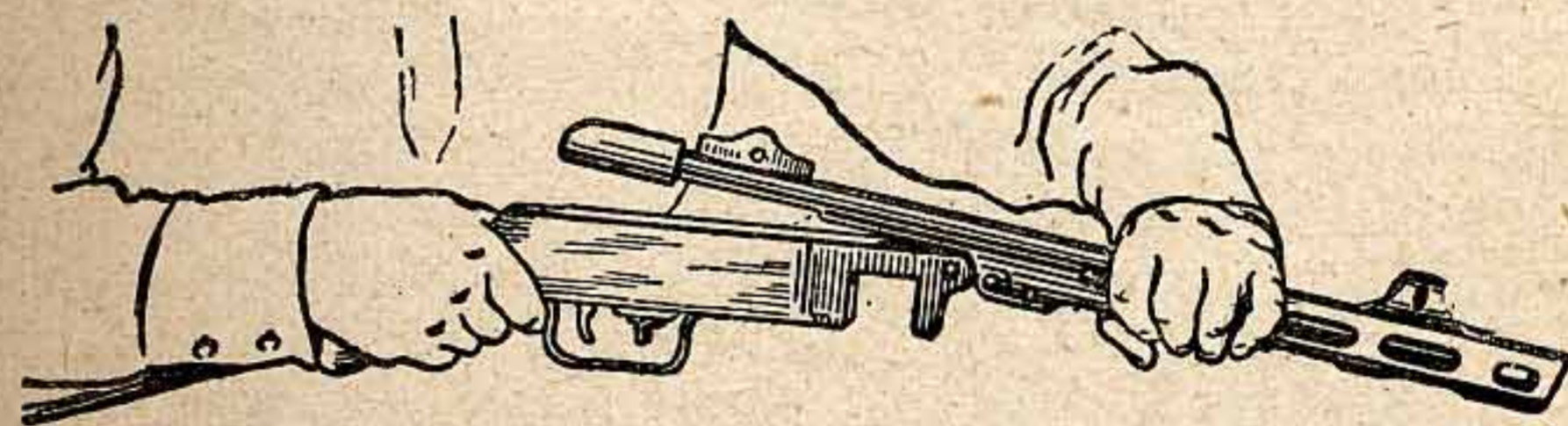
Рис. 38. Как отделить ствольную коробку от затворной
