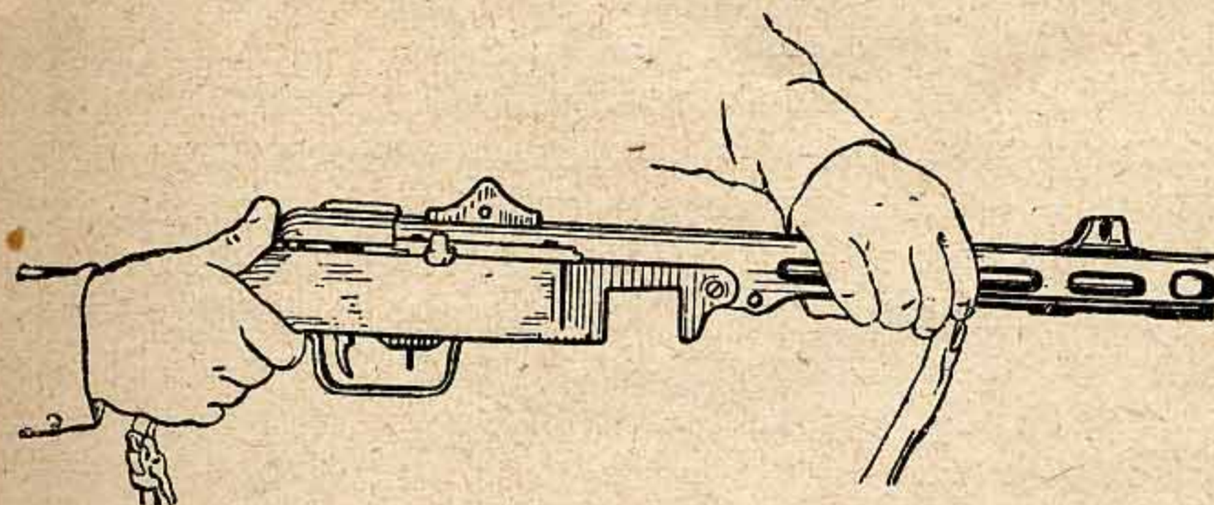
Рис. 31. Как открыть затворную коробку
