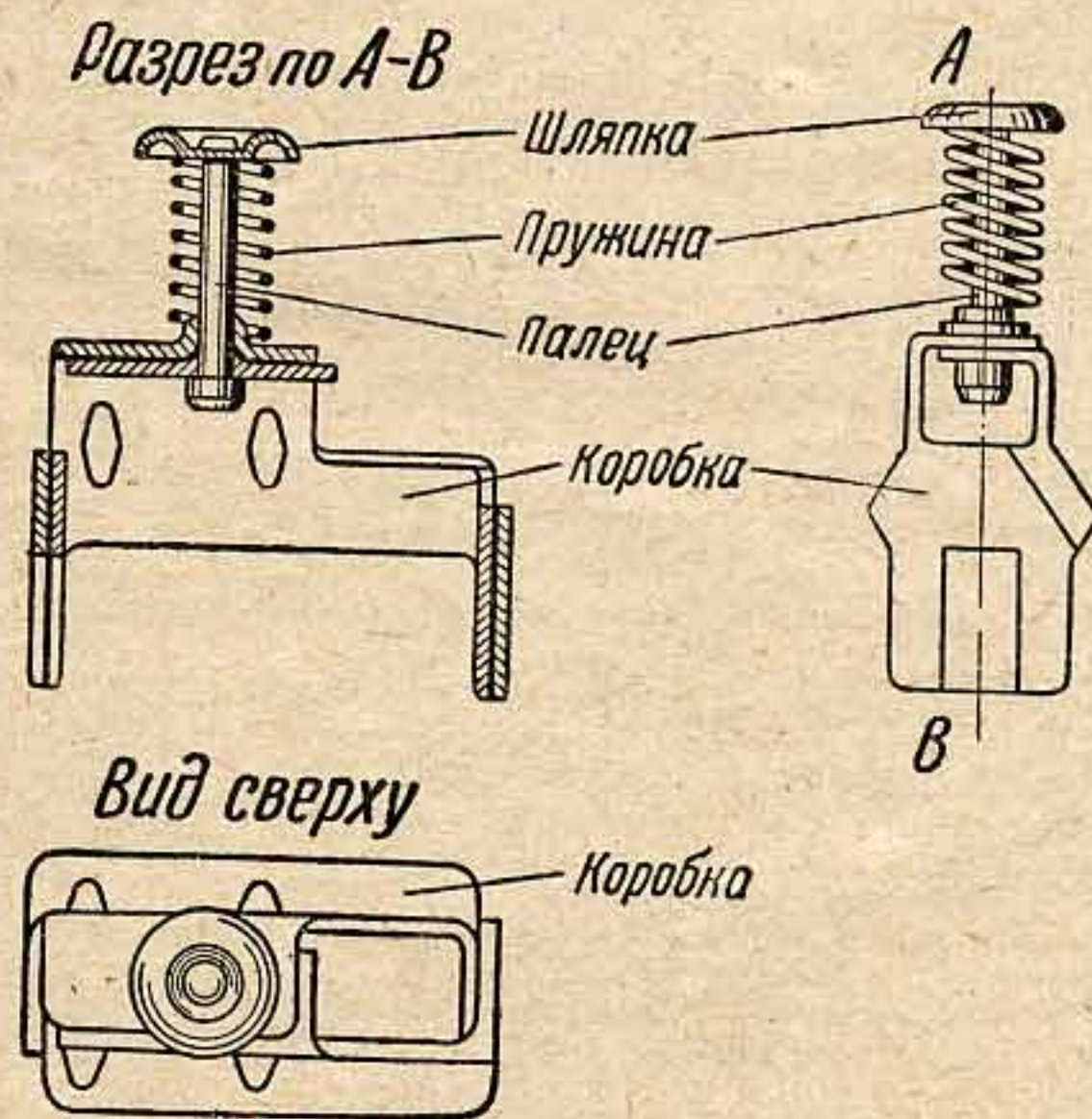
Рис. 58. Приспособление для снаряжения коробчатого магазина
