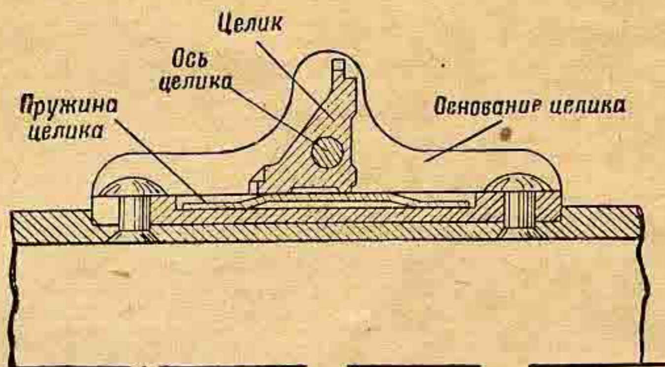
Рис. 6. Прицел с вращающимся целиком
