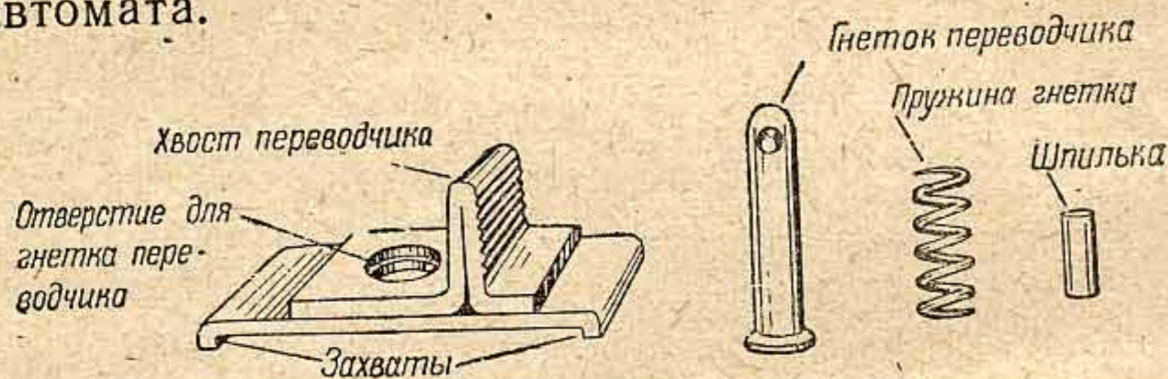
Рис. 15. Гнеток переводчика
