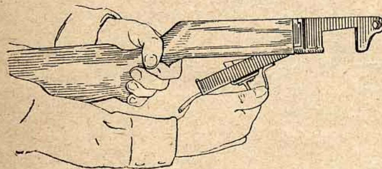
Рис. 42. Как отделить спусковую коробку от ложи
