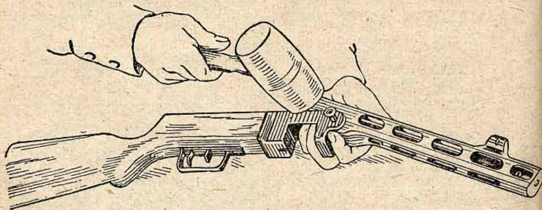
Рис. 51. Как вставить соединительную ось
