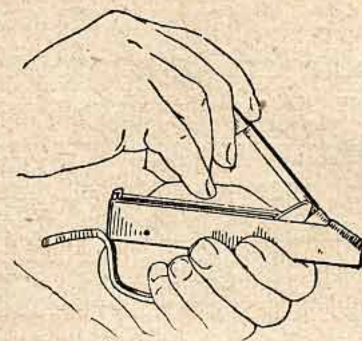
Рис. 46. Как вынуть спусковой рычаг
