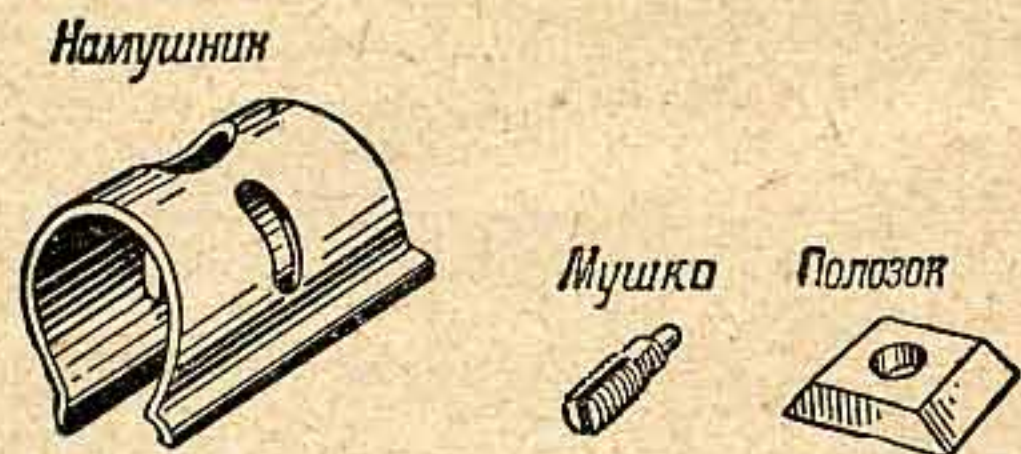
Рис. 4. Мушка
